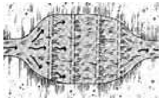
Esquema de un ensanchamiento de cauce formando una poza de sedimentación // Fuente: Medina, 1991
