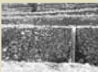
Canales de desagüe en terrazas Fuente: Cusichaca Trust
