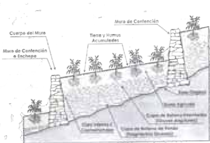
Configuración y partes de una terraza precolombina. Fuente: Chilon, 2009
