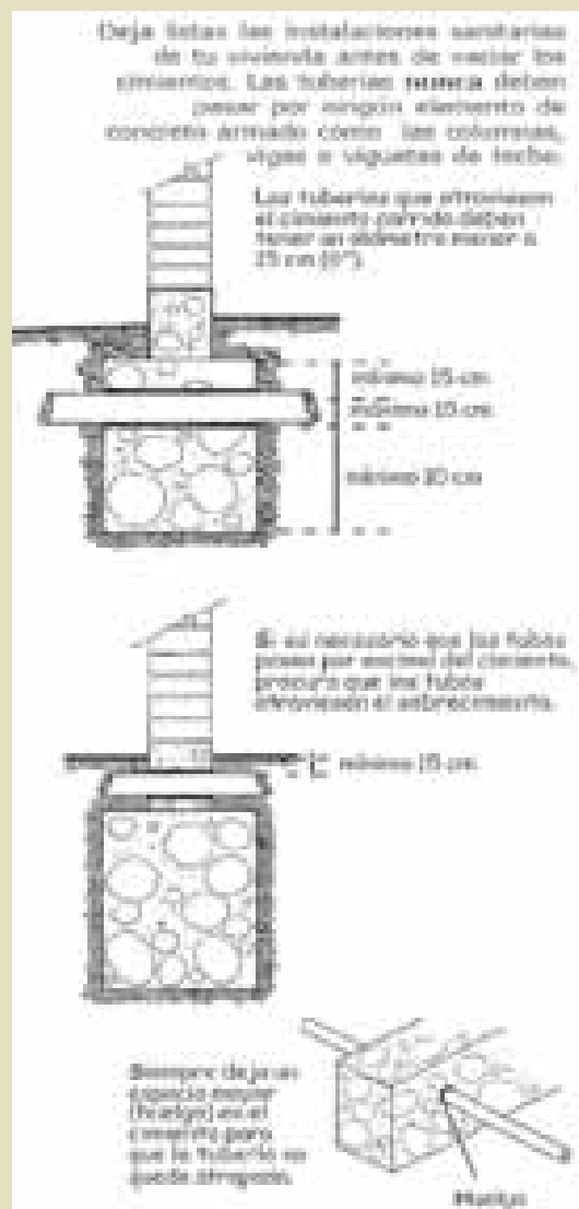
Instalaciones sanitarias Fuente: M. Blondet (PUCP y SENCICO), 2005
