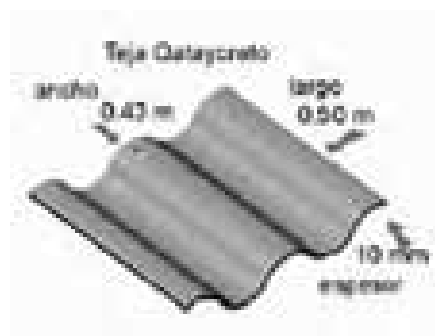
Teja de concreto // Fuente: Soluciones Prácticas
