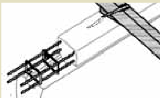
Amarre de vigüeta a viga solera Fuente: CENAPRED
