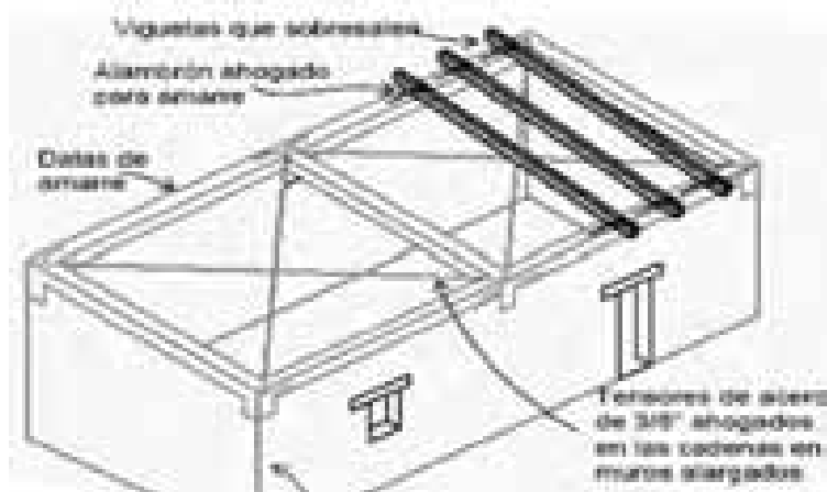
Sistemas de amarres en techos. // Fuente: CENAPRED
