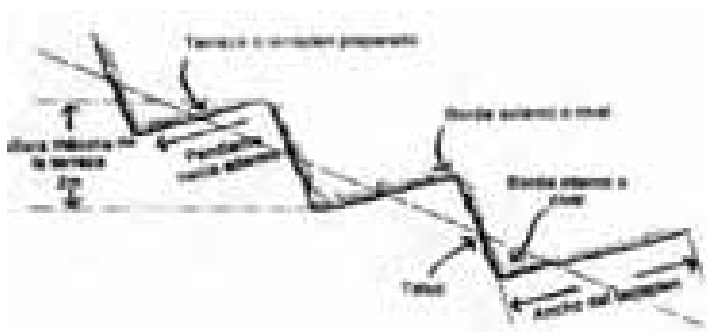
Esquema de una terraza de banco // Fuente: Medina, 1991
