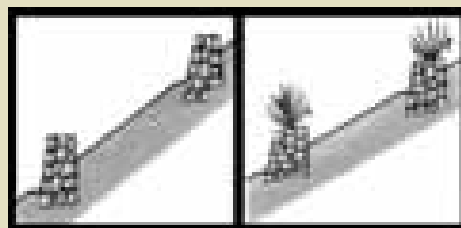
Izquierda: Terraza de formación lenta con muros de piedra. Derecha: terraza de formación lenta con muros de piedra y barreras vivas
