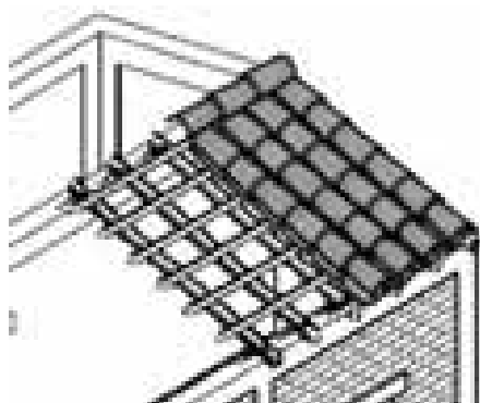
Colocación de tejas // Fuente: CENAPRED
