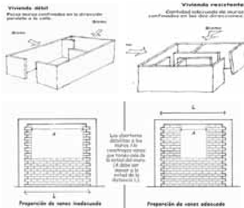
Algunos criterios de diseño a considerar al construir Fuente: M. Blondet (PUCP y SENCICO), 2005
