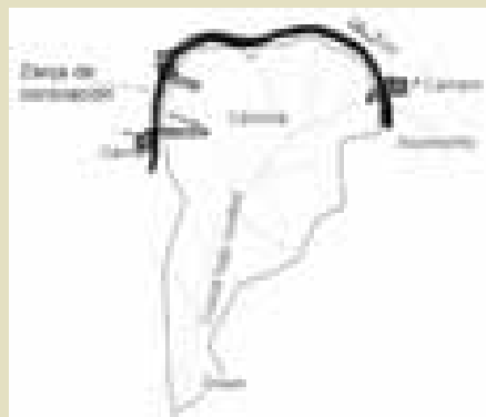
Representación de la zanja de coronación en una cárcava. Las áreas cuadradas indican las cámaras donde llega el agua concentrada por las zanjas // Fuente: Promic, FAO
